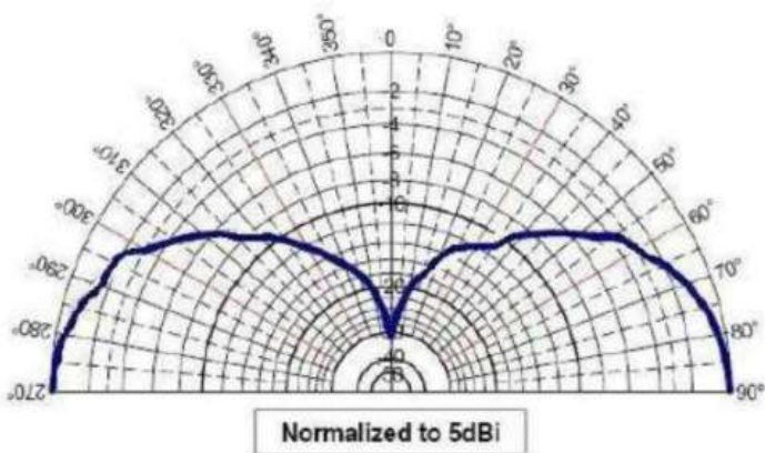
Elevation Pattern (Z, Y or H-Plane)
